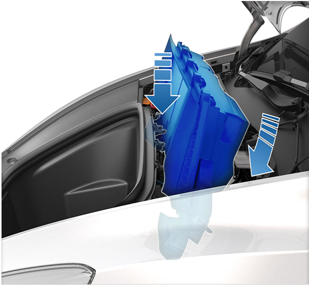
b. 10mm 소켓으로 볼트(2개)를 조이고 5Nm(3.7ft-lb) 토크로 조입니다.
