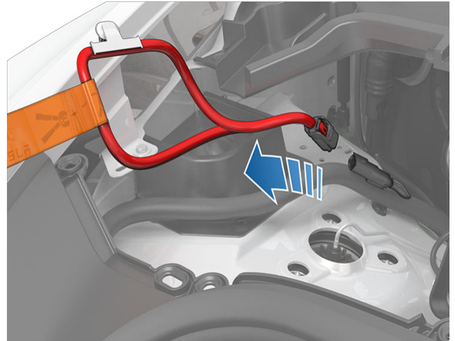
7. 10mm 소켓으로 단자 커버를 분리하고 양극(+) 단자 클램프를 납산 배터리의 양극(+) 포스트에 고정하는 너트를 풀습니다. 양극(+) 포스트에서 단자 클램프를 분리하고 단자 클램프를 마른 천으로 닦습니다.
