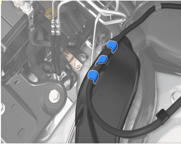
c. 10mm 소켓으로 HEPA 필터 어셈블리를 차량에 고정하는 볼트(2개)를 탈거합니다.
