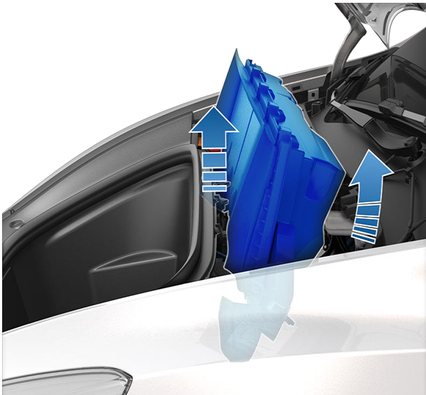
d. 필터 어셈블리의 후면 가장자리가 브레이크액 저장 탱크를 지나도록 위로 기울여 차량에서 HEPA 필터 어셈블리를 탈거합니다. 다른 구성품에 부딪히거나 손상을 주지 않도록 주의하면서 필터 어셈블리를 차량에서 들어 올려 빼냅니다.
