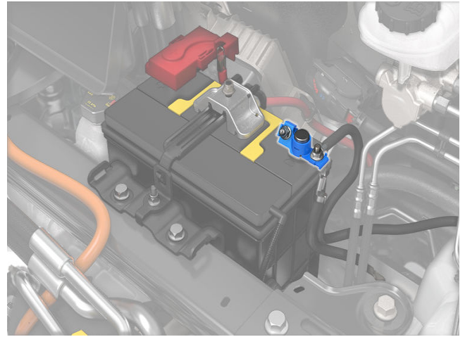
6. 적색 잠금 탭을 본인을 향해 밀면서 검은색 탭을 눌러 응급구조대 루프를 연결 해제합니다.
