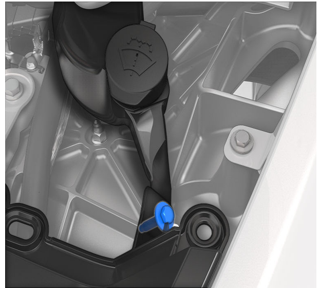
e. 10mm 소켓을 사용하여 워셔액 저장 탱크 넥을 후드 내 보관 유닛에 고정하는 볼트를 장착합니다. 볼트를 5Nm(3.7ft-lb) 토크로 조입니다.
