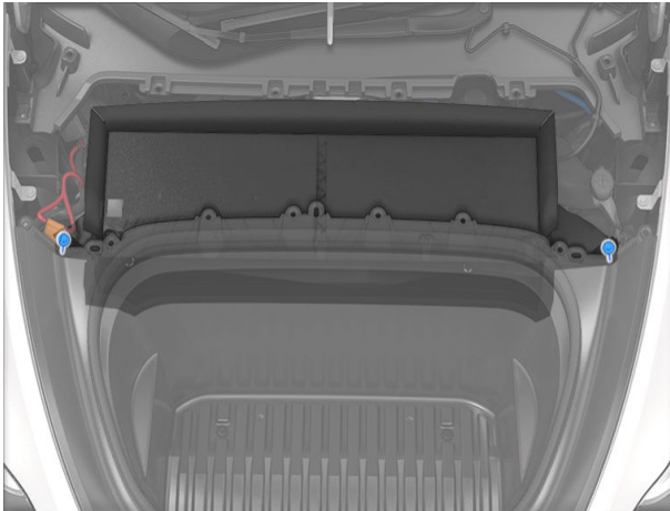
d. 필터 어셈블리의 후면 가장자리가 브레이크액 저장 탱크를 지나도록 위로 기울여 차량에서 HEPA 필터 어셈블리를 탈거합니다. 다른 구성품에 부딪히거나 손상을 주지 않도록 주의하면서 필터 어셈블리를 차량에서 들어 올려 빼냅니다.
