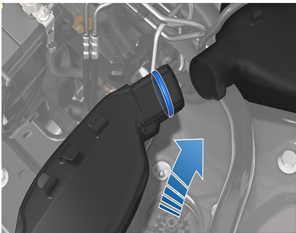
d. 호스가 탭으로 고정되도록 배치합니다.
