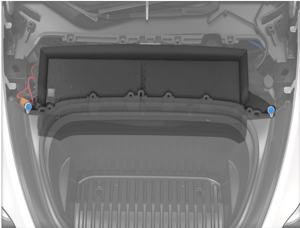
c. 워셔 탱크 넥의 O링이 완전히 안착했는지 확인한 다음, 워셔 탱크 넥을 워셔 탱크에 삽입하여 장착합니다.
