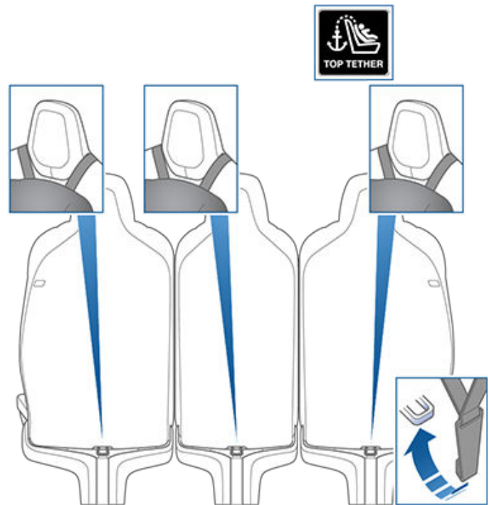
Cinghie di stabilizzazione doppie - Sedili a panchetta della seconda fila
