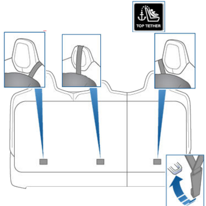
Cinghia di stabilizzazione singola - Sedili terza fila
